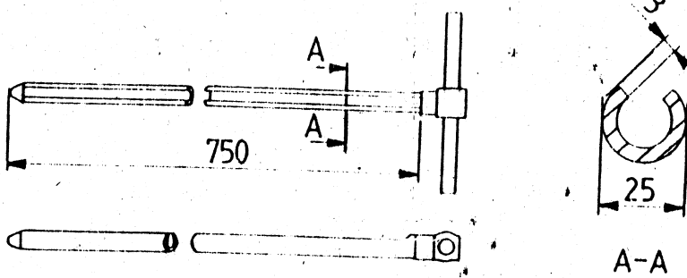
Hình 3; Ống lấy mẫu kín đầu
