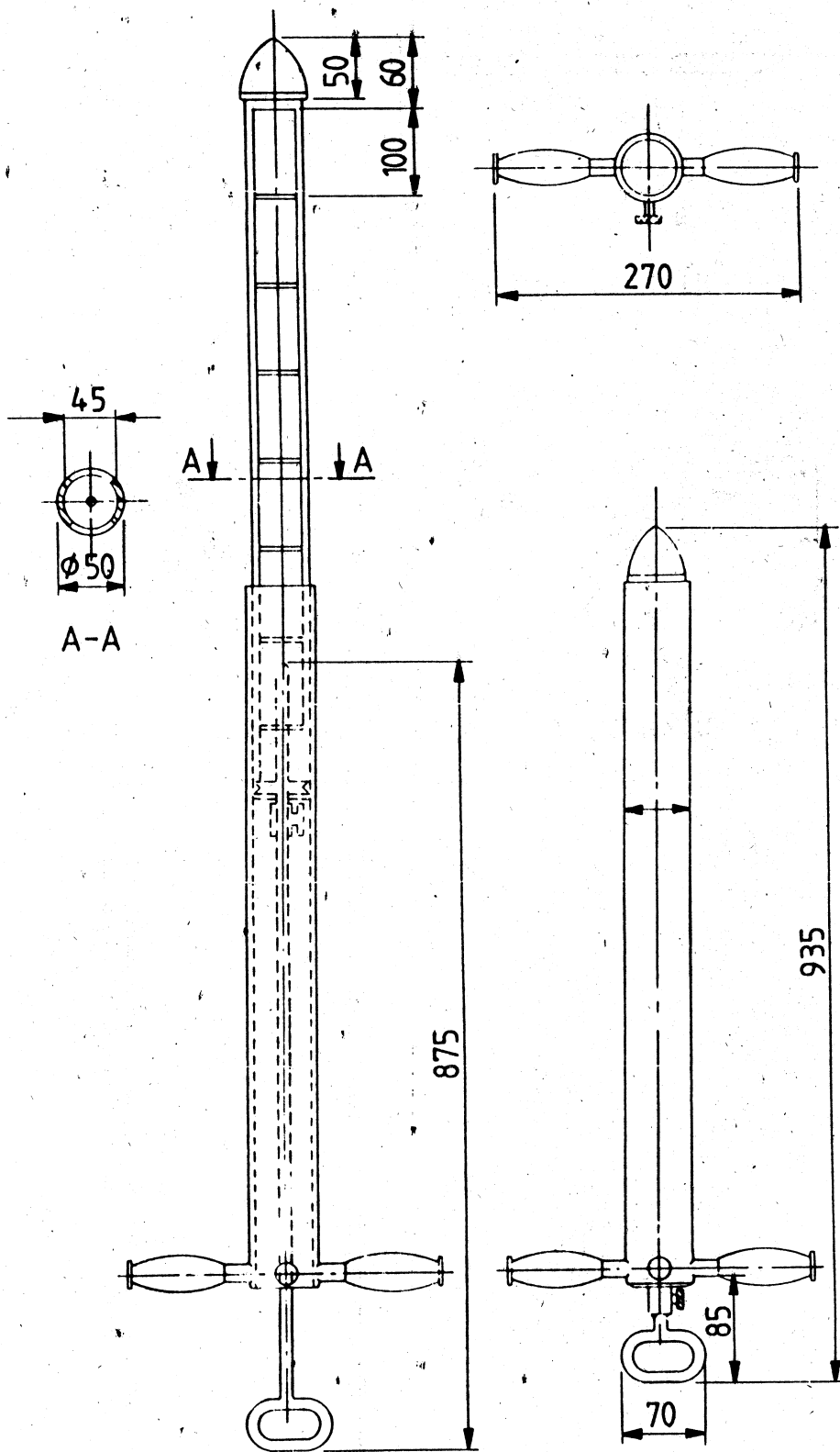
Hình 5. Ống lấy mẫu
