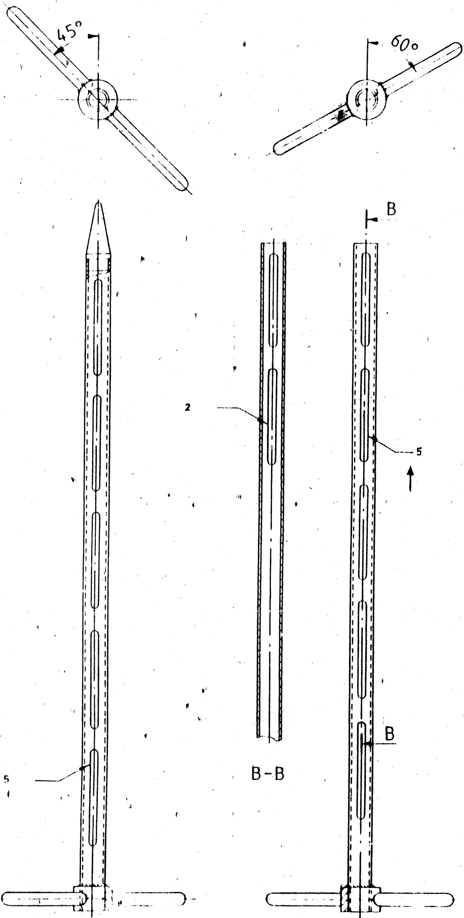
Hình 6. Ống lấy mẫu
