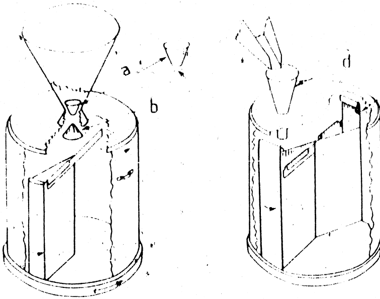
Hình 10. Cái chia mẫu quay
