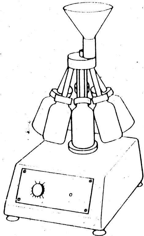
Hình 12. Máy chia mẫu quay
