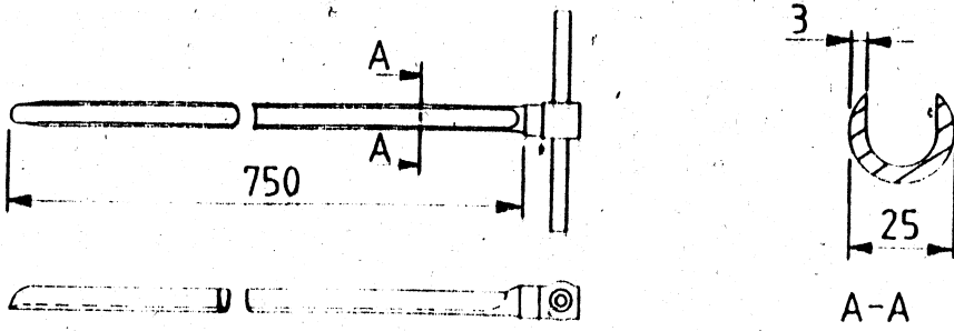
Hình 2. Ống lấy mẫu hở đầu
